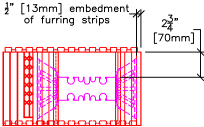
ELEVATION B-B
