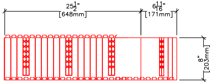
ELEVATION A-A
