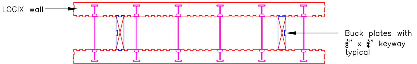
SECTION A-A
