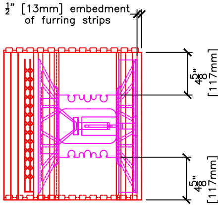
ELEVATION B-B
